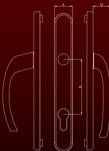
Shutter door handle
